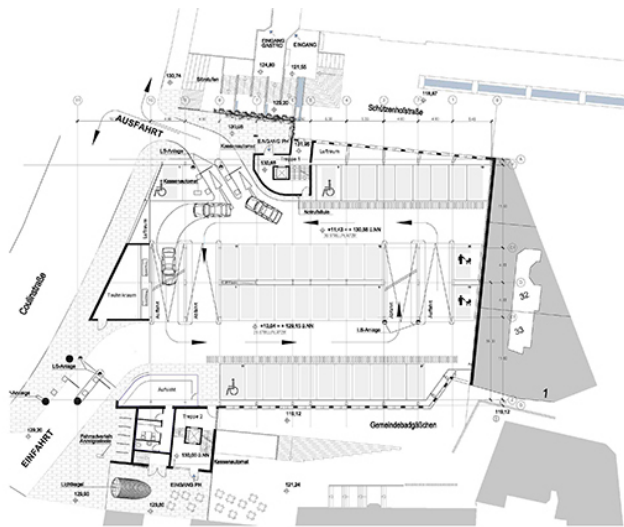
Grundriss 3. Obergeschoss Ein- und Ausfahrt
