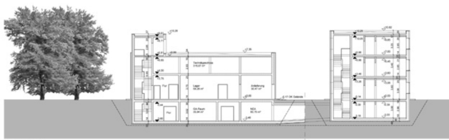
SCHNITT A-A
