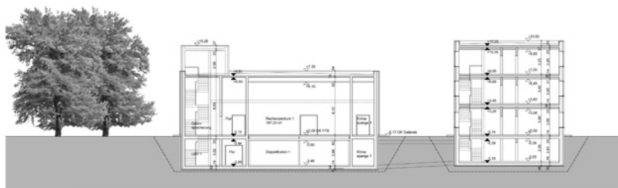
SCHNITT B-B
