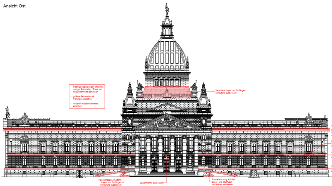
Ansicht Ost
