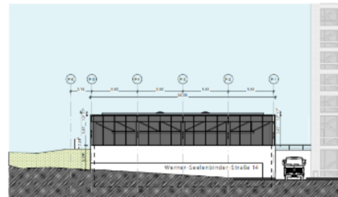
Ansiht Nord
