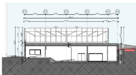
Schnitt CC: Nebeneingang
