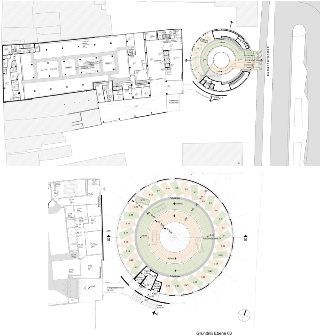
Grundriß Ebene 03
