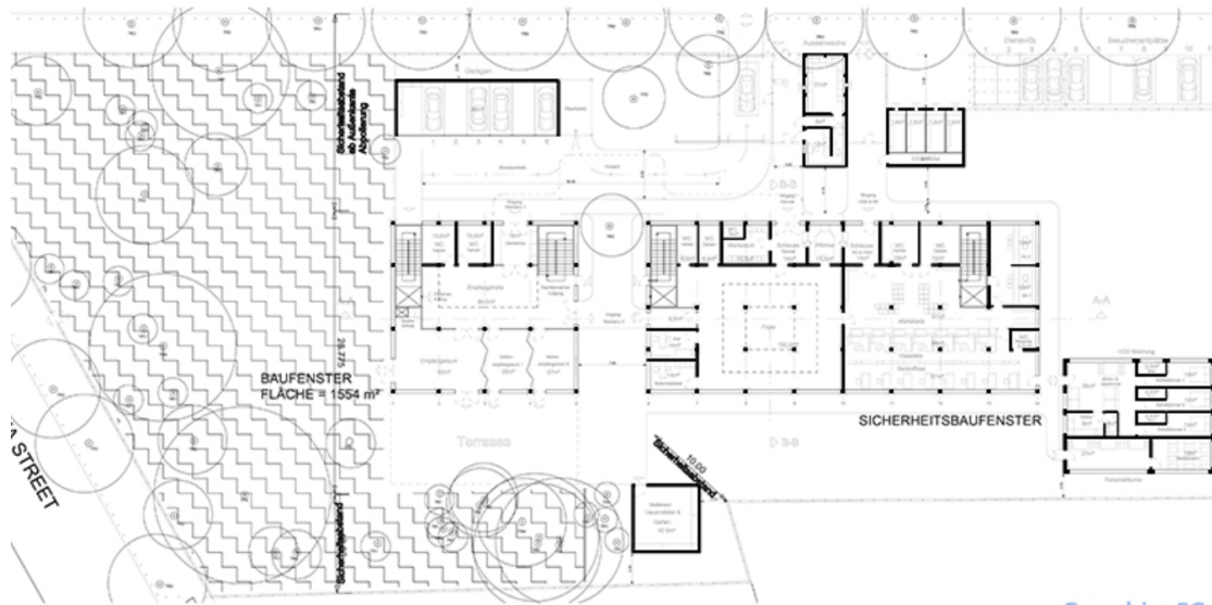
Grundriss EG
